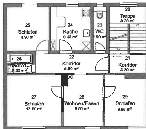
1. Obergeschoss - 1:100
