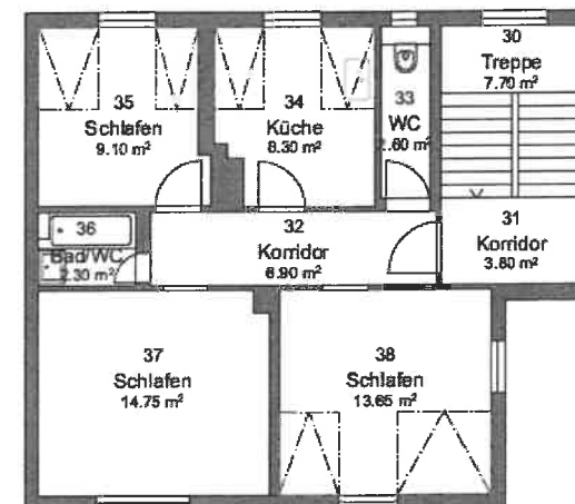
Dachgeschoss - 1:100
